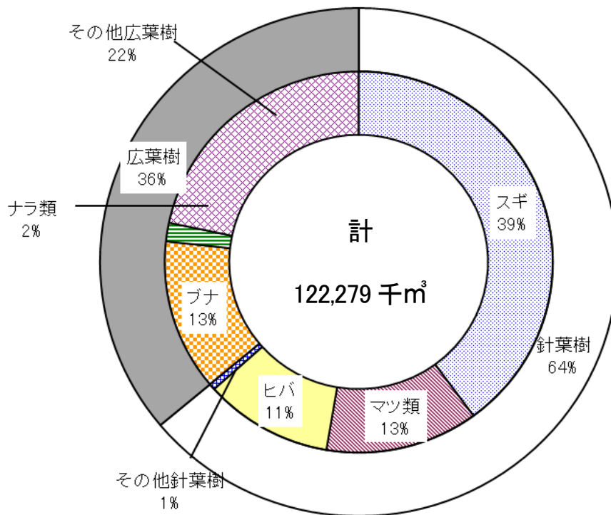
図7 樹種別蓄積（平成30年4月1日現在）
