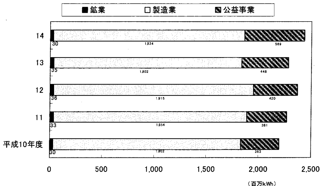
図11 大口電力産業別需要量の推移
