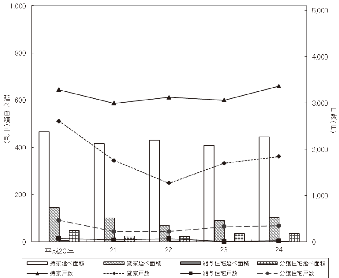
図10 利用関係別着工新設住宅の推移
