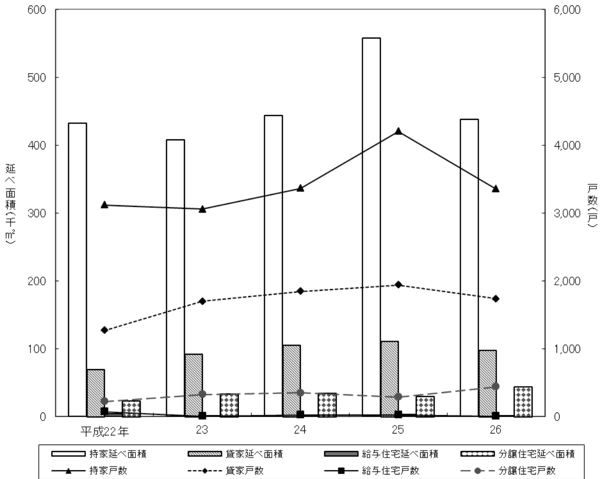
図10 利用関係別着工新設住宅の推移
